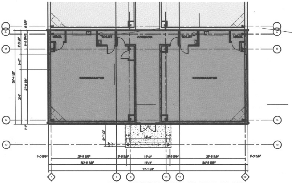
03 - DIMENSIONED FLOOR PLAN SCALE: 1/8" = 1'-0"
