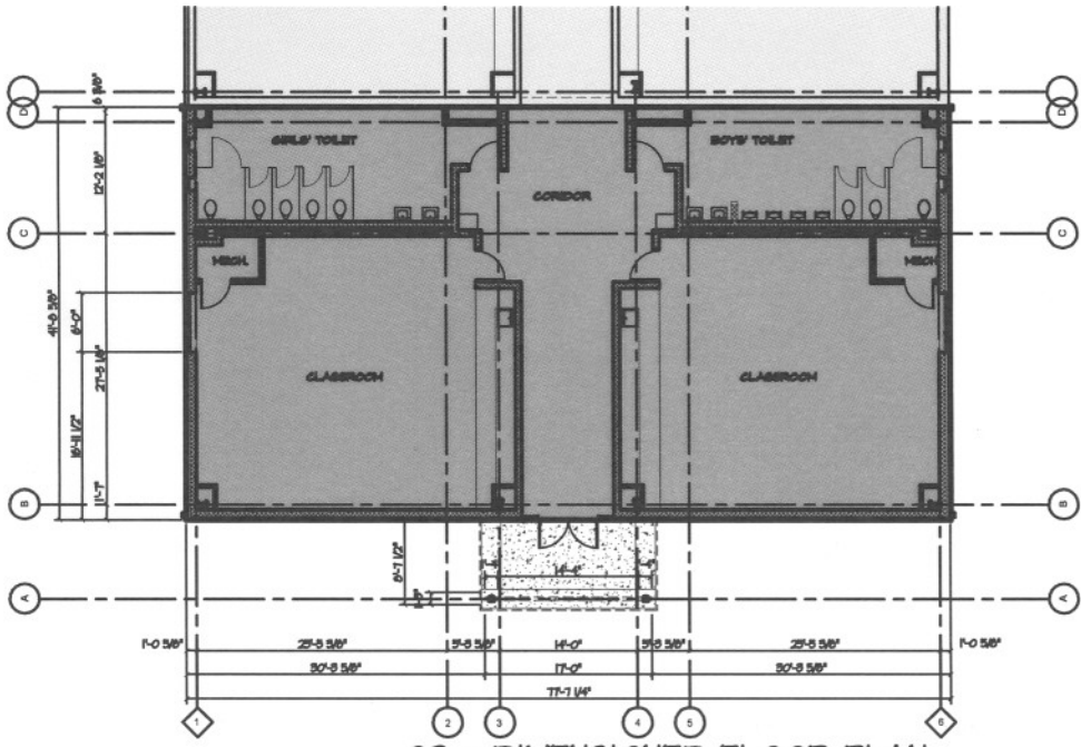
02 - DIMENSIONED FLOOR PLAN SCALE: 1/8" = 1'-0"
